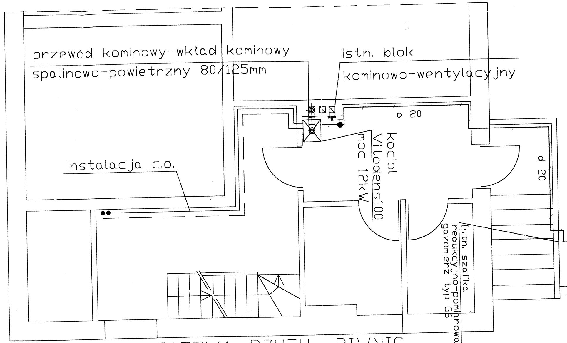
INSTALACJA GAZOWA RZUTU PIWNIC skala 1:50
