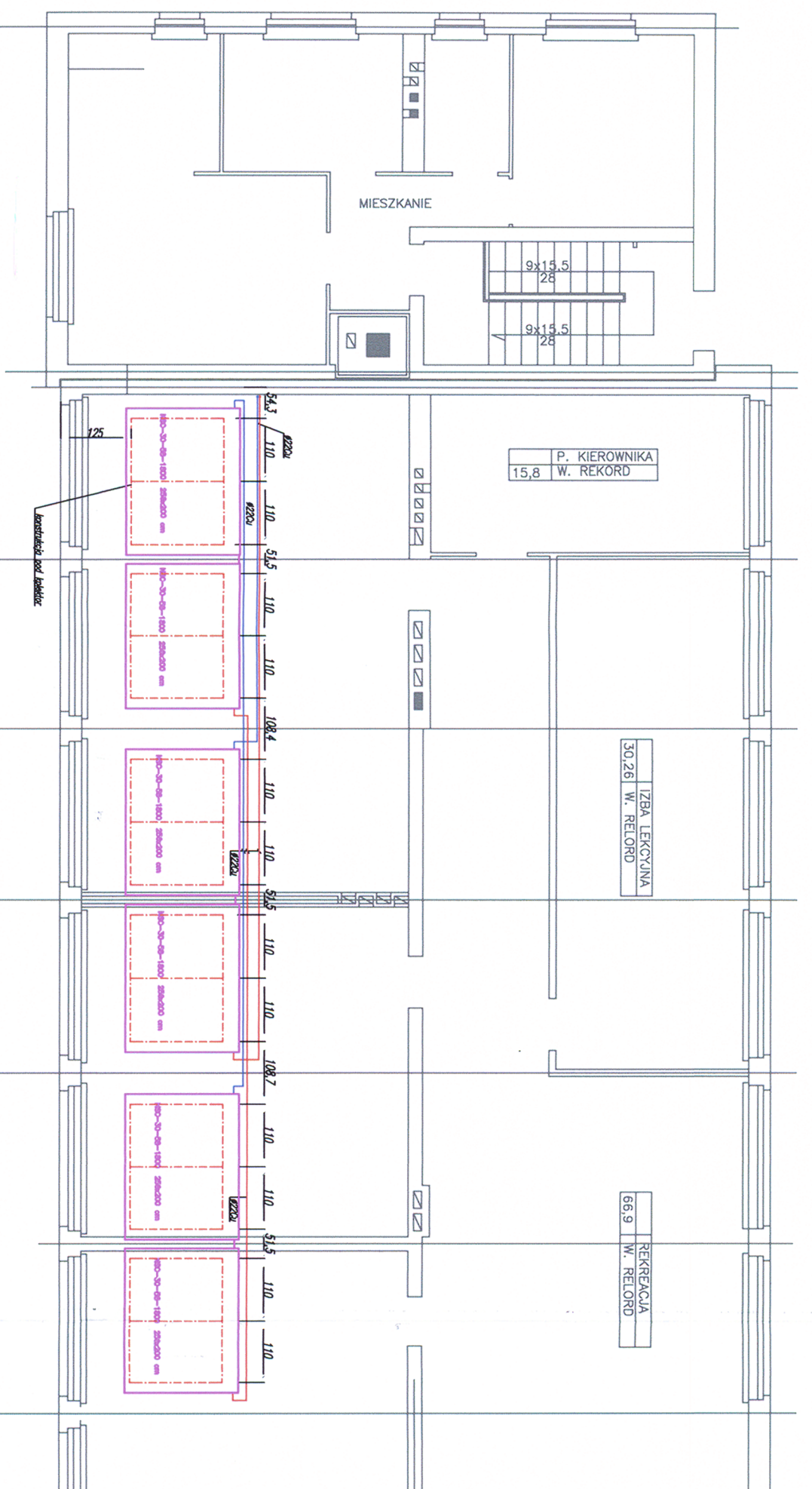
RZUT PIĘTRA 1:100
