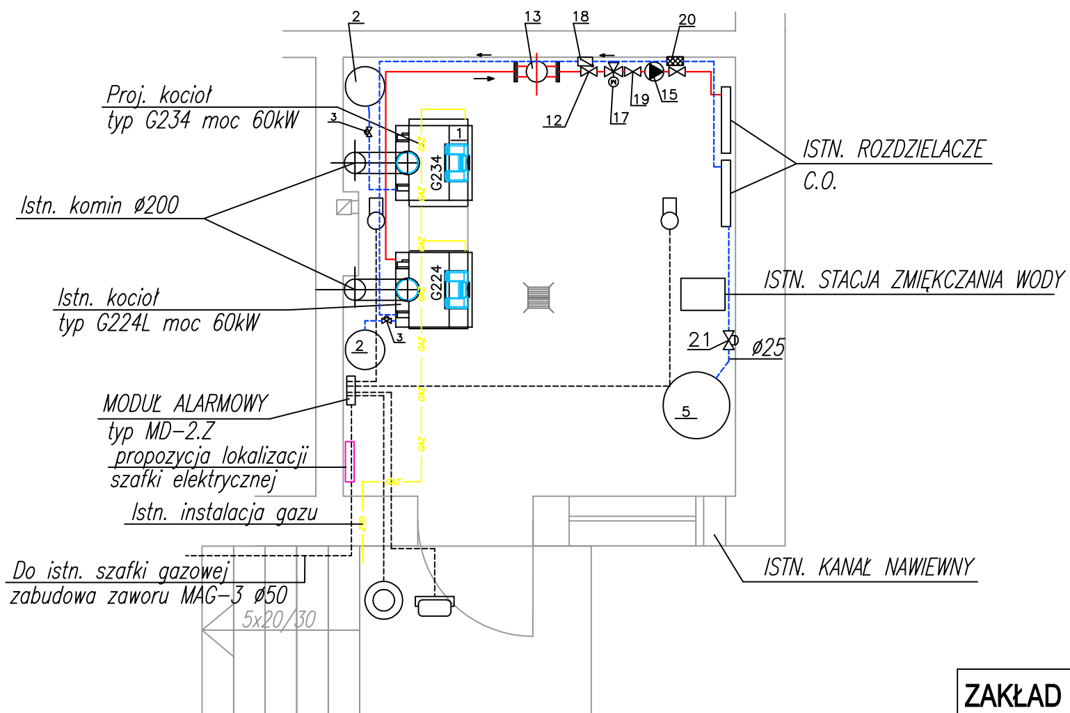
Rzut kotłowni
