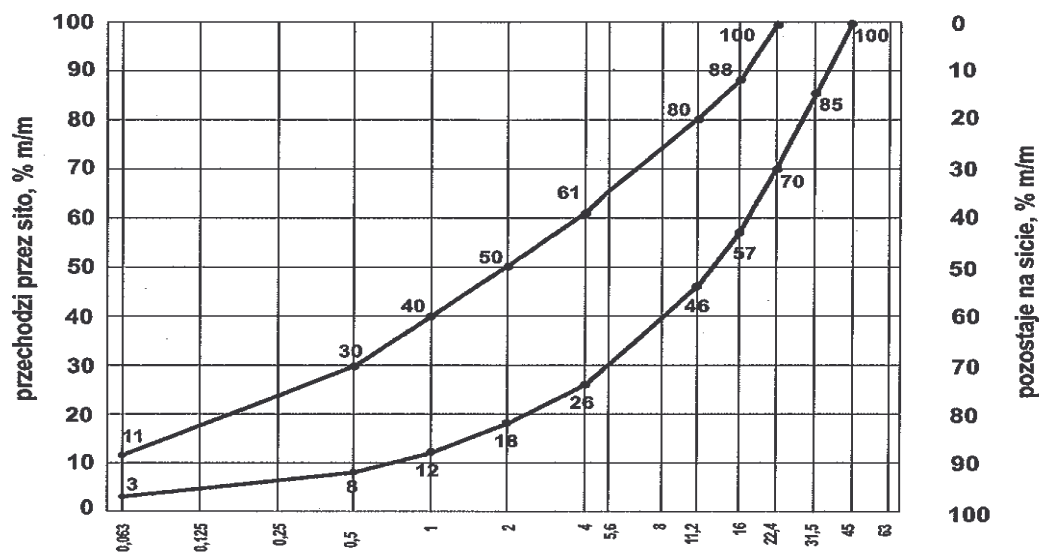
Rys.1 Uziarnienie mieszanki CBGM 0/31,5
