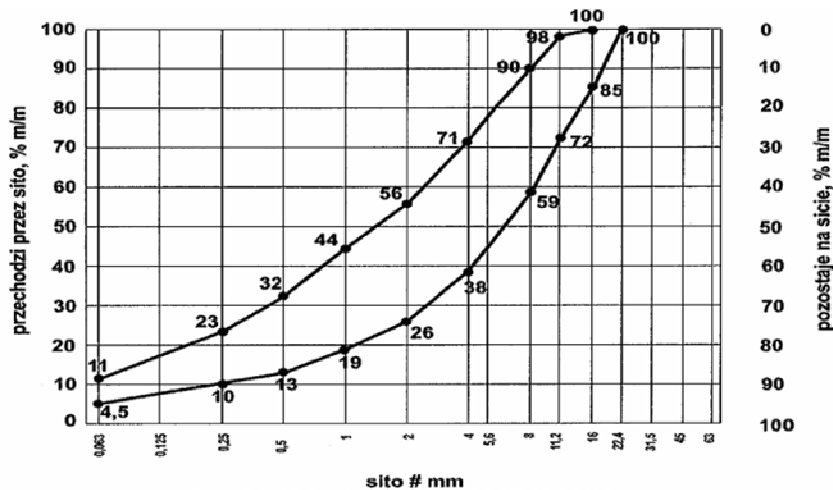
Rys.3 Uziarnienie mieszanki CBGM 0/16
