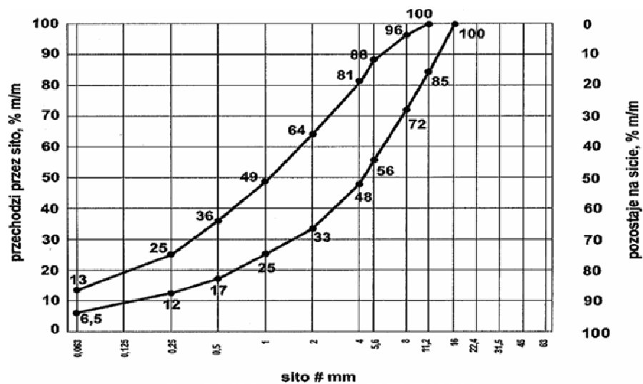
Rys.4 Uziarnienie mieszanki CBGM 0/11,2
