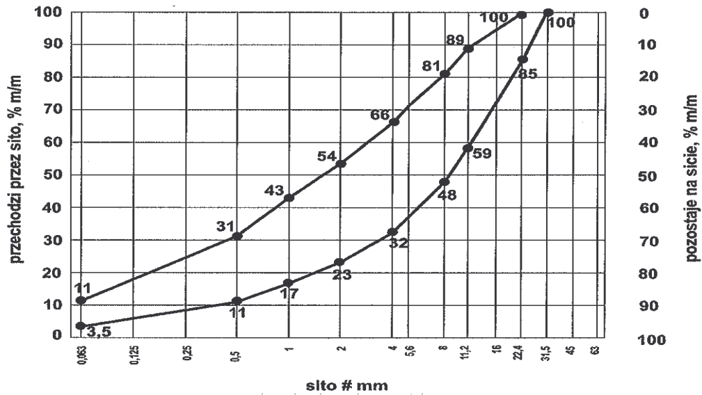
Rys.2 Uziarnienie mieszanki CBGM 0/22,4
