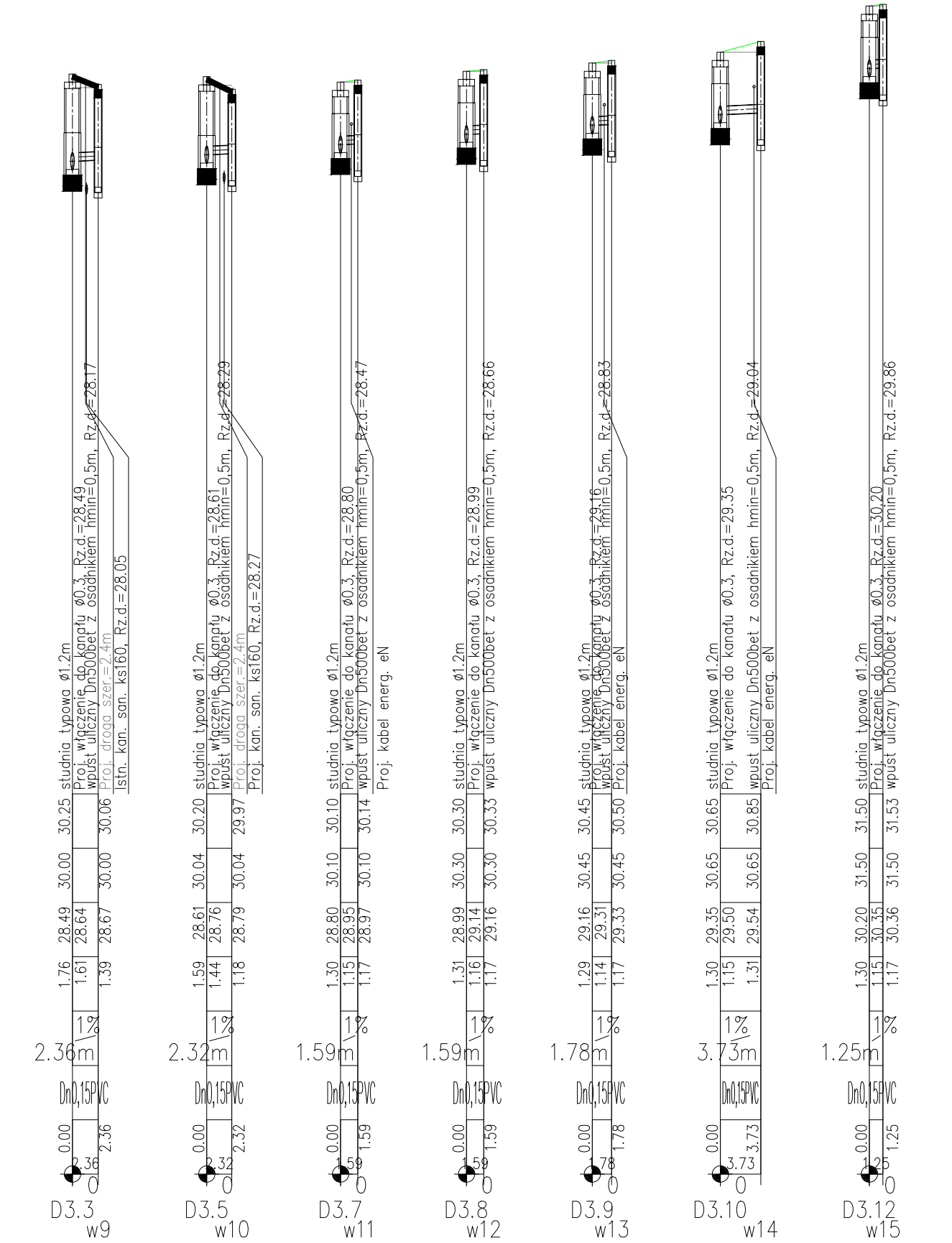
PROFILE PODŁUŻNE KANAŁÓW - WYLOT W3
