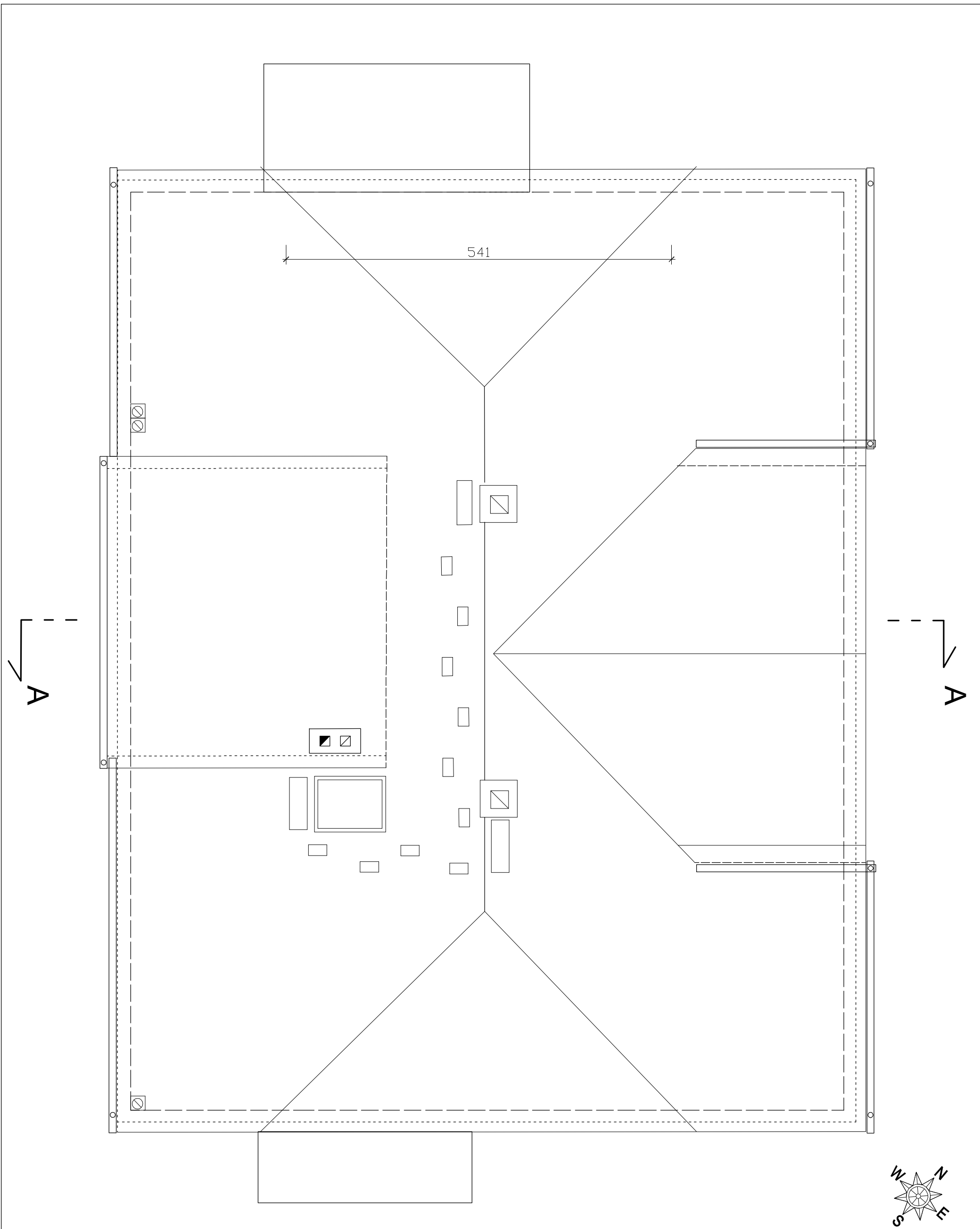
RZUT DACHU Skala 1:50
