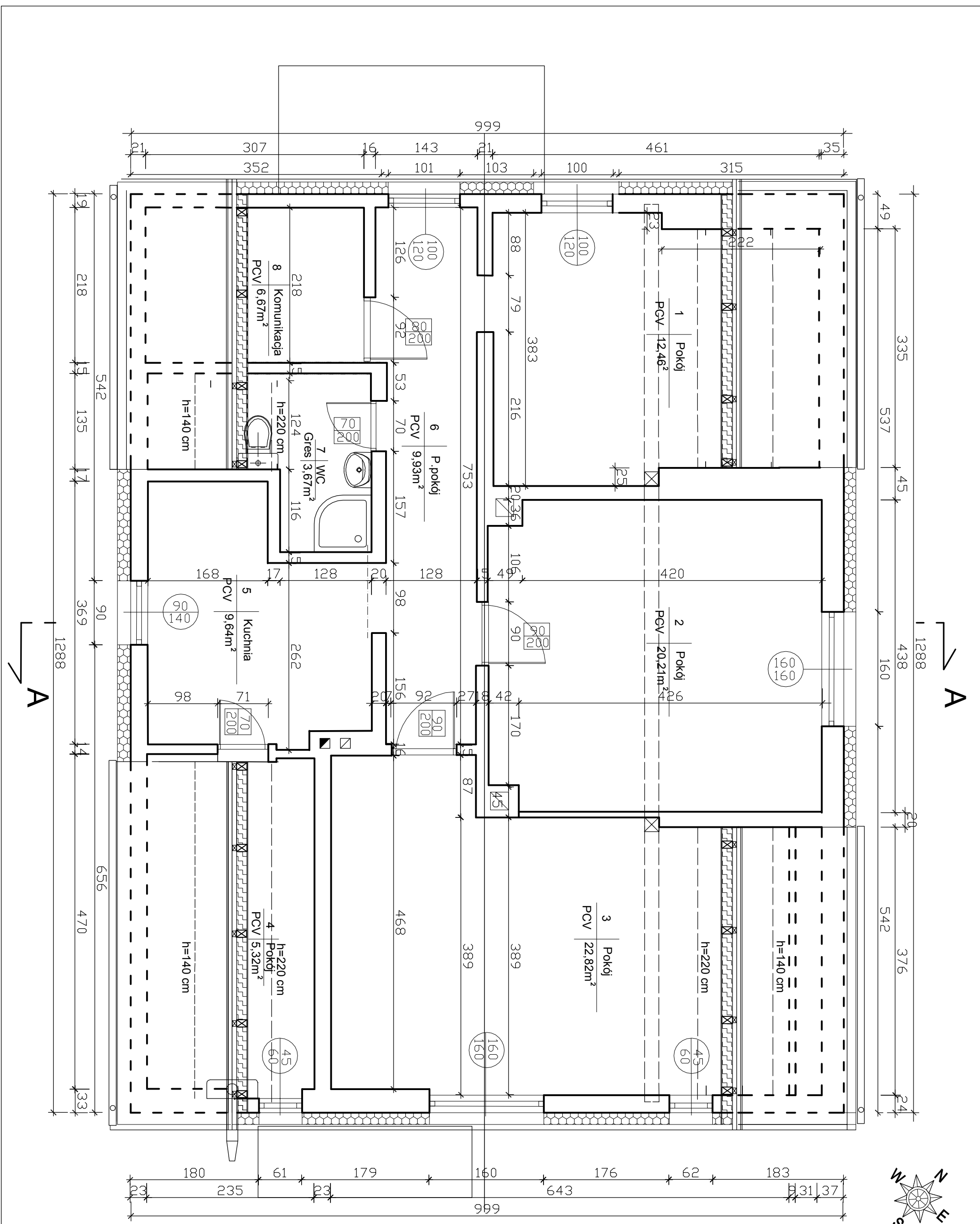
RZUT PODDASZA Skala 1:50
