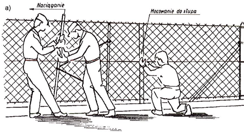
Rys. 9. Przykłady mocowania siatki do linek usztywniających (wg [6])
