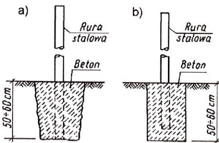
Rys. 4. Przykład ustawiania słupków ogrodzenia (wg [6]) a) Ustawianie „na oko”, b) Ustawienie „pod sznur”, c) Sprawdzanie odchylenia słupka od pionu
