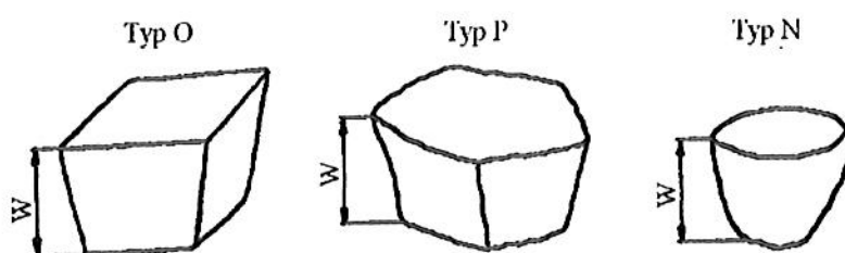
Tablica 2. Wymiary i dokładność wykonania brukowca wg PN-B-11104 [11]
