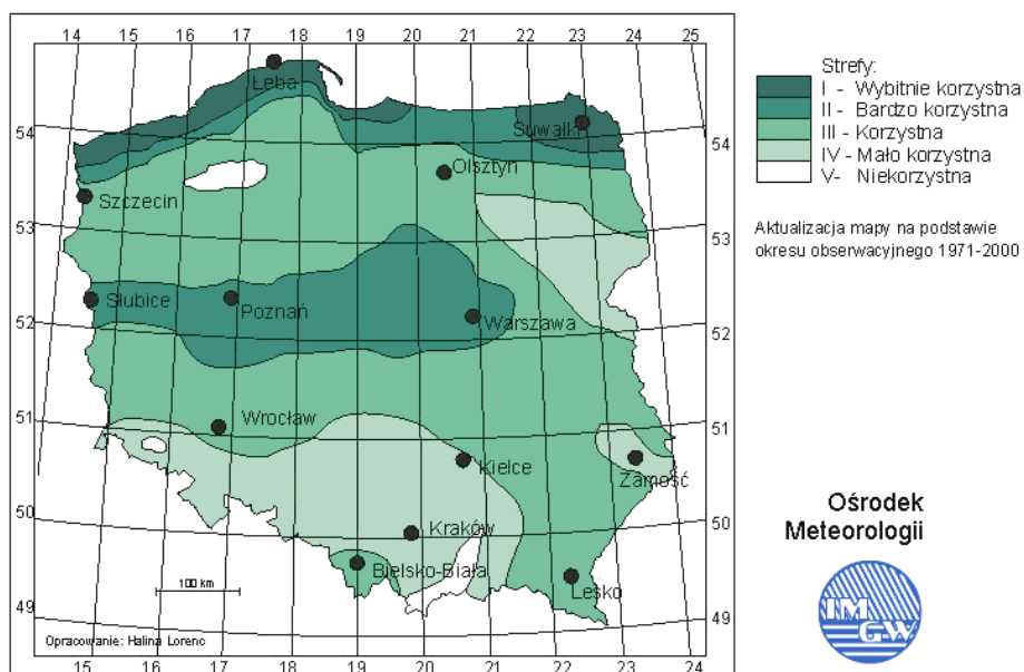
Ryc. 5. Strefy energetyczne wiatru w Polsce
